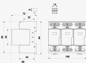
Rozměry
