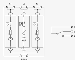
Schéma zapojení
