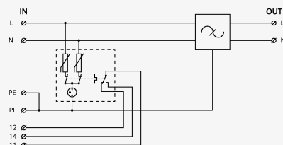
Schéma zapojení
