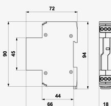
Rozměry
