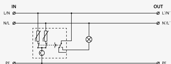
Schéma zapojení
