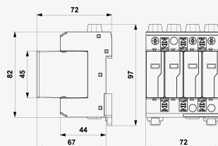
Rozměry
