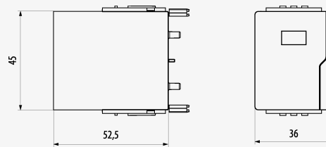
Produktabmessungen
