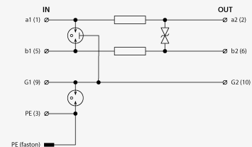
Prinzipschaltbild
