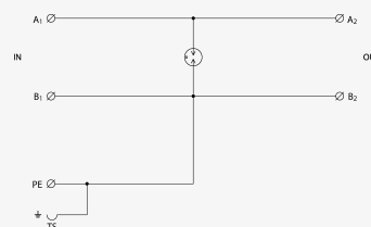
Prinzipschaltbild
