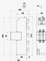
Produktabmessungen
