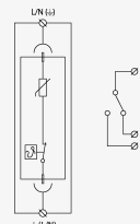
Schéma zapojenia
