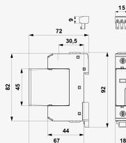
Rozmery produktu
