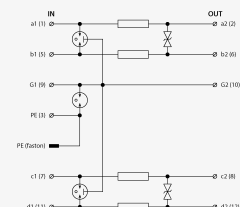
Schéma zapojenia
