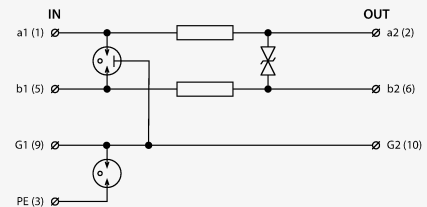
Schéma zapojenia
