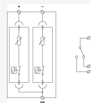
Schéma zapojenia
